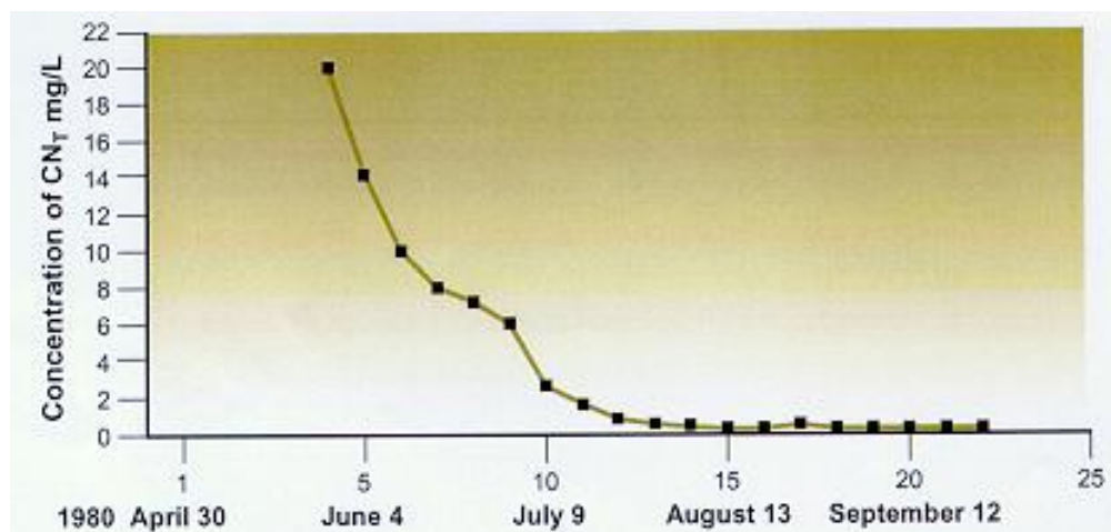
Figura 5. Ejemplo de degradación de Cianuro en diques de colas someros Fuente: adaptado de Schmidt et al., 1981
