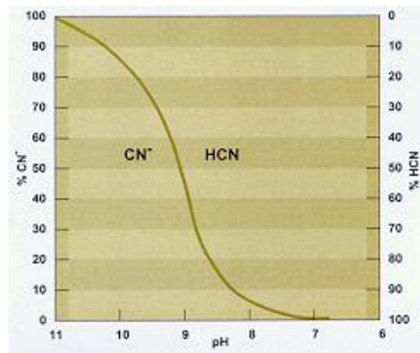
Figura 3: Equilibrio de pH entre \text{CN}^-/\text{HCN}
